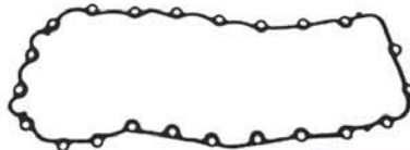
Junta de carter 22 agujeros
